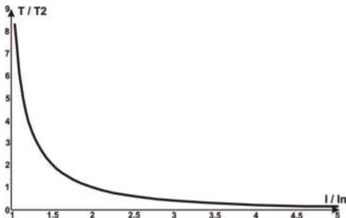
Рисунок 6 – Токо-временная характеристика
